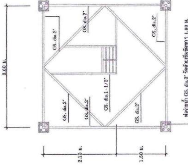
แปลนชั้นที่ 3 ขนาดเส้น 1 : 50
